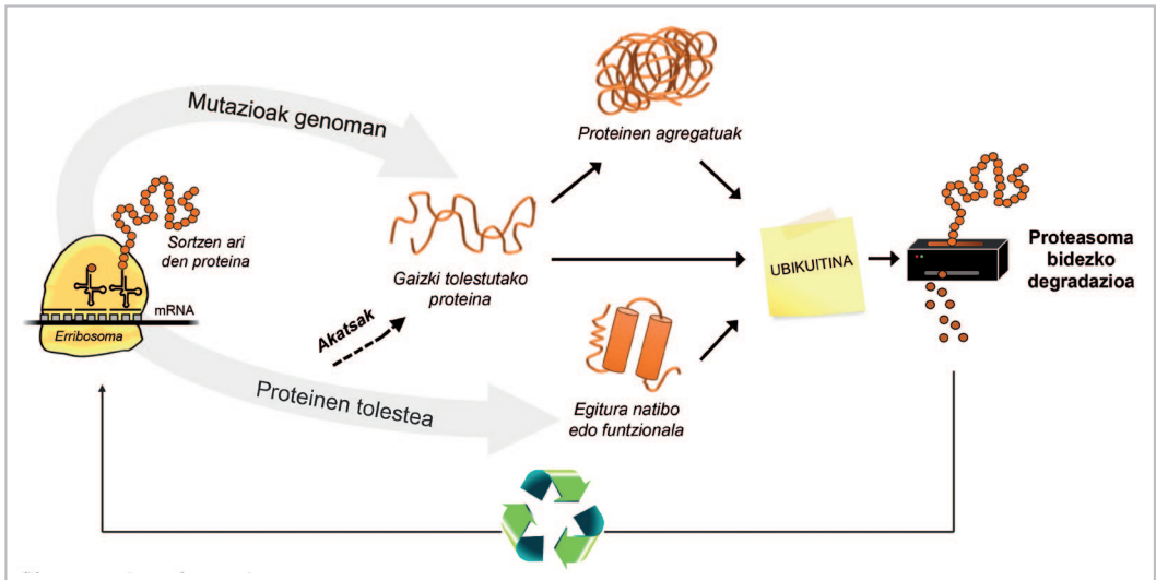
3. irudia. Zelula osasuntsuetako proteinen "bizi-zikloa". Oro har, proteinak eta jada zelularentzat beharrezkoak ez diren proteinak ubikitinarekin markatzen dira, proteasoma bidez degradatzeko. Prozesu horretan askatzen diren aminoazidoak proteina berriak ekoizteko berrerabil daitezke.
